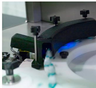
Las botellas se marcan en su parte inferior; el escudo de protección del láser se muestra en negro.
