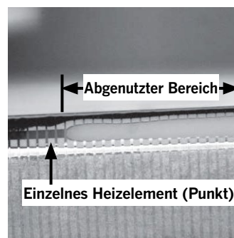
Gebrochene Heizelemente (Punkte) verursacht durch Abrieb, der die Schutzschicht des Druckkopfs abgetragen hat
