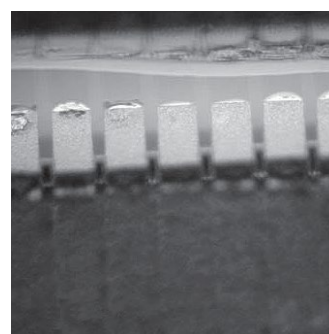
Nahaufnahme beschädigter Heizelemente (Punkte), die zu leeren Stellen im Druckbild führen
