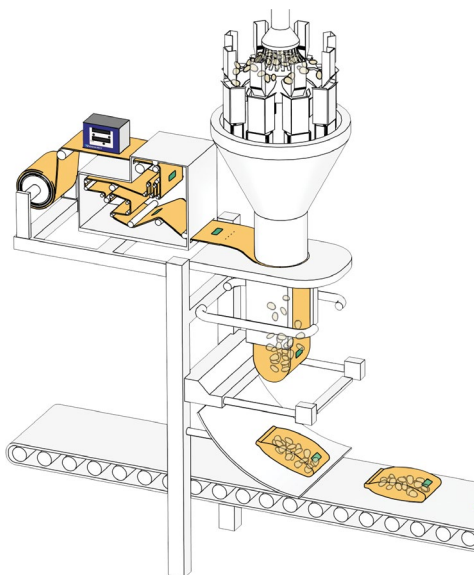
Beispiel für DataFlex® mit Vertikal-Schlauchbeutel-Verpackungsmaschine
