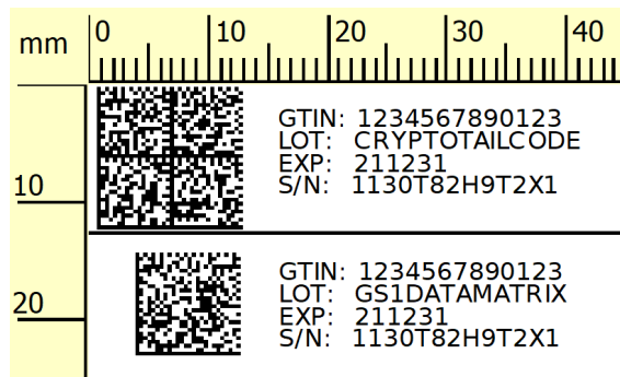
符号尺寸为 36x36 模块的典型加密编码（顶部）与常见的符号尺寸为 26x26 模块的 GS1 DataMatrix 码（底部）的比较。
