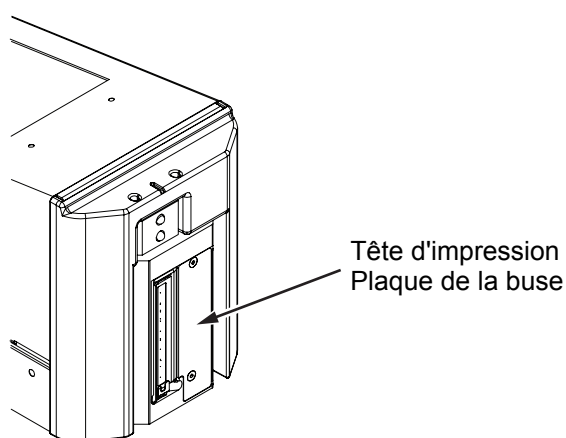
Figure 4-21 : Plaque de buse de tête d'impression -Videojet 2350
