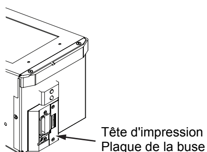
Figure 4-20 : Plaque de buse de tête d'impression -Videojet 2340
