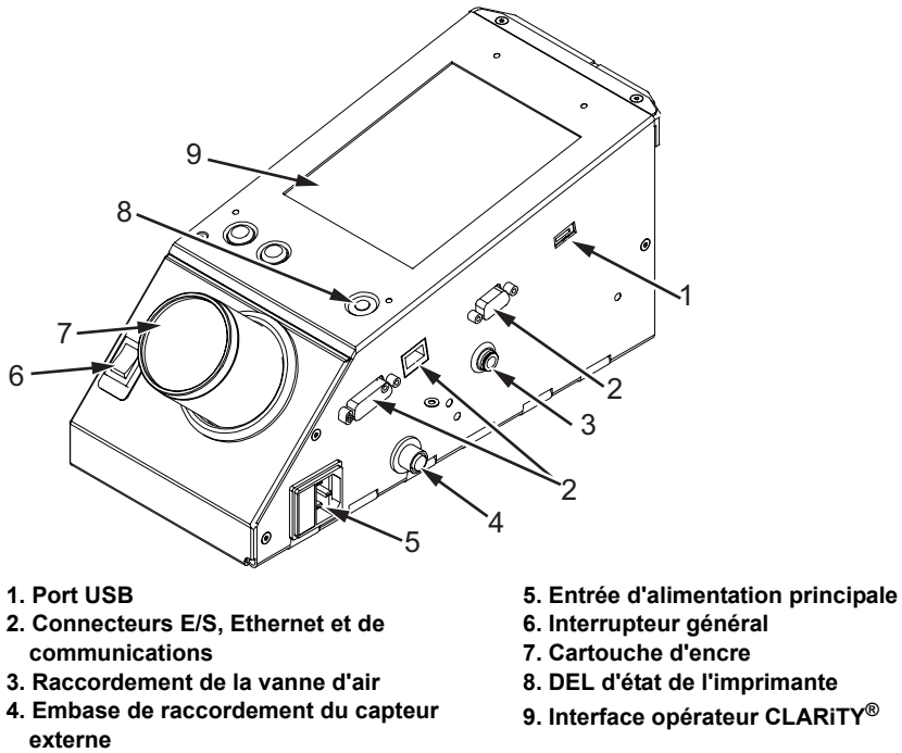
Figure 1-1 : Pièces d'imprimante - Videojet 2340
