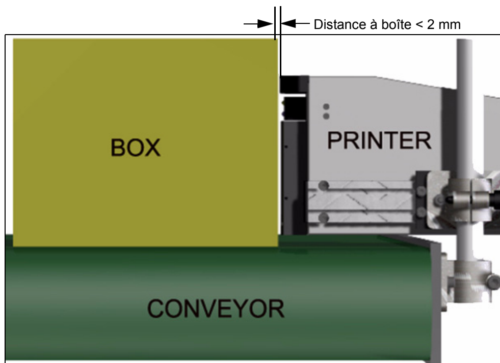
Figure 4-17 : Distance à boîte
