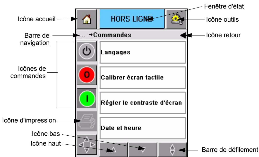
Figure 3-2 : Icônes de raccourci
