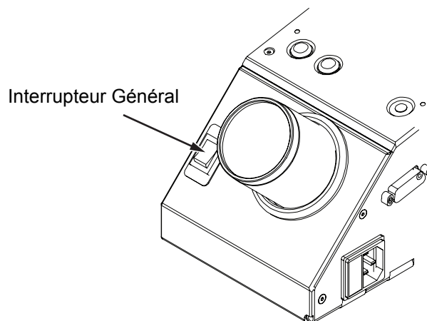
Figure 4-1 : Interrupteur Général - Videojet 2340
