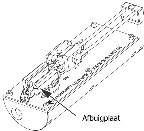
Afbeelding 6-7: De afbuigplaat reinigen (Videojet 1650 UHS- 50 micron)
