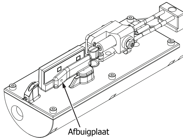
Afbeelding 6-6: De afbuigplaat reinigen (Videojet 1650 )
