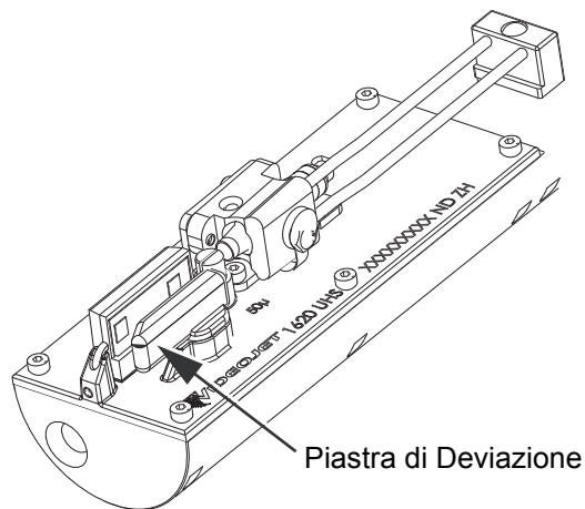
Figura 6-5: Pulizia della piastra di deviazione
