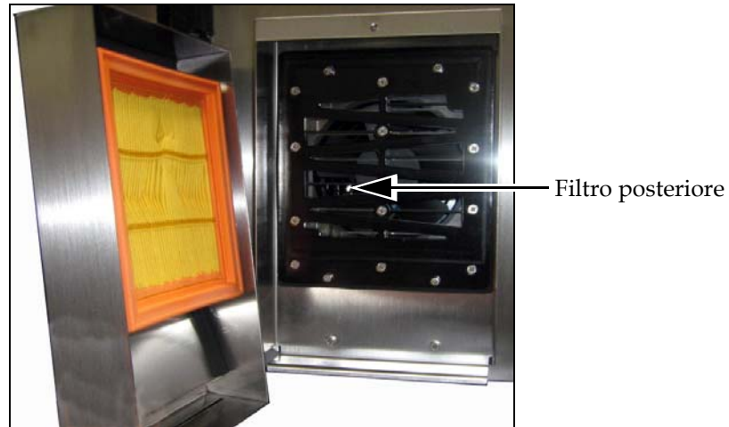
Figura 3-10: Filtro posteriore (Versione IP65)
