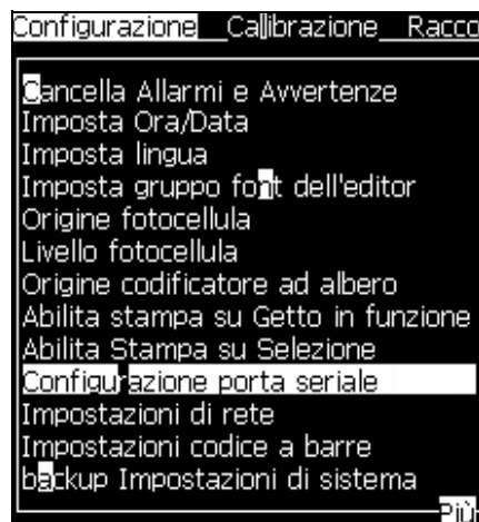
Figura 4-20: Menu Configura
