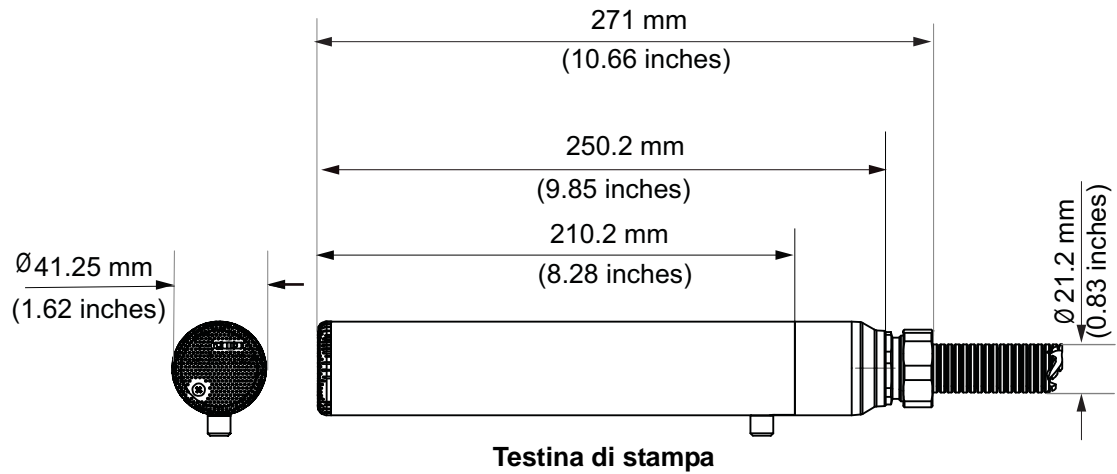
Figura A-2: Dimensioni della stampante (continua)
