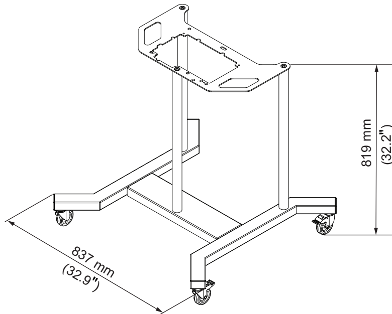
Afbeelding A-2: Mobiel printerstatief
