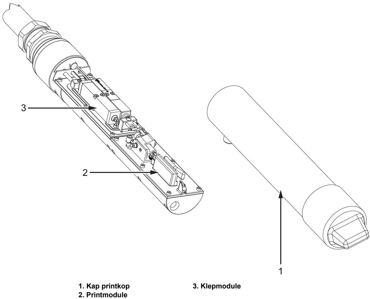
Afbeelding 3-12: Printkopoverzicht
