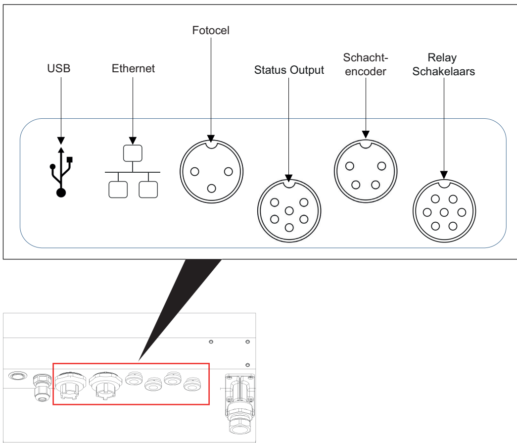
Afbeelding 3-11: Standaard IO
