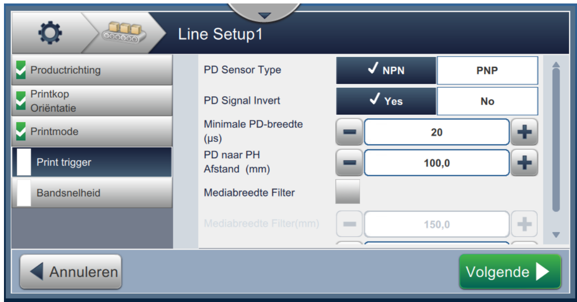
Afbeelding 6-32: Lijninstelling - Printrigger
