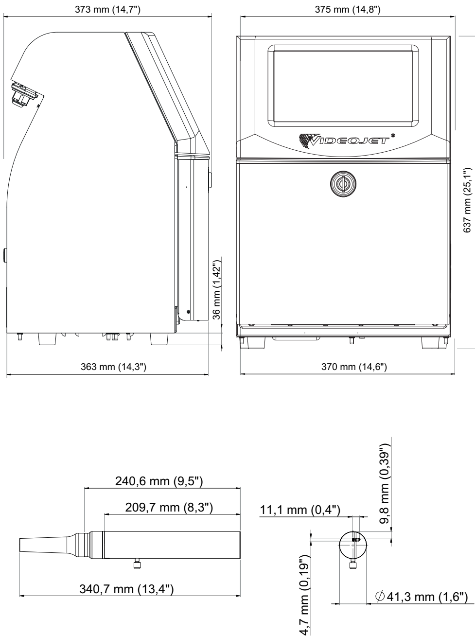
Afbeelding A-1: Printerafmetingen
