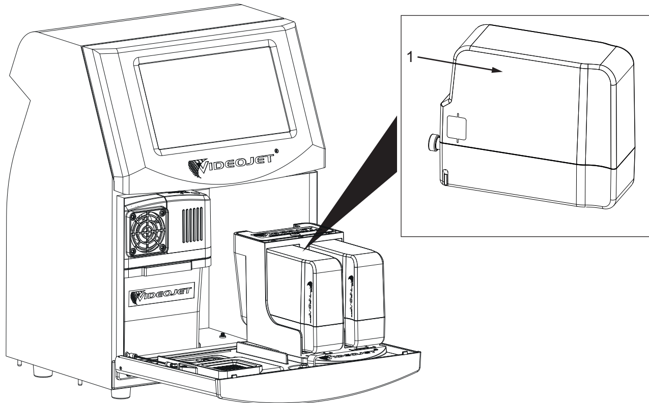
1. Vloeistofcartridge
