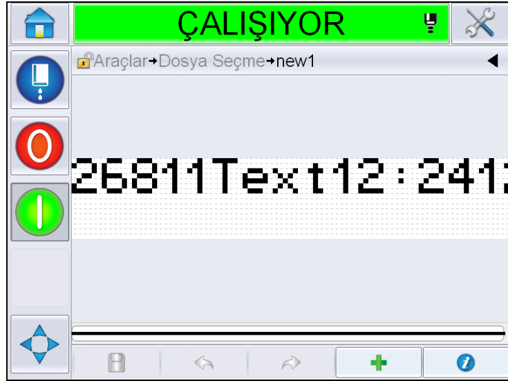
Şekil 5-41: Mesaj Sayfası
