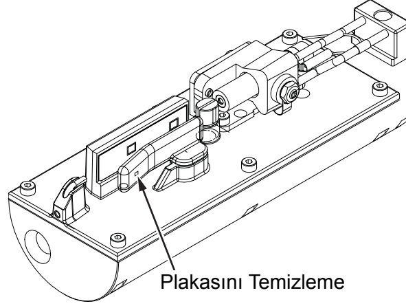
Şekil 6-5: Saptırma Plakasını Temizleme
