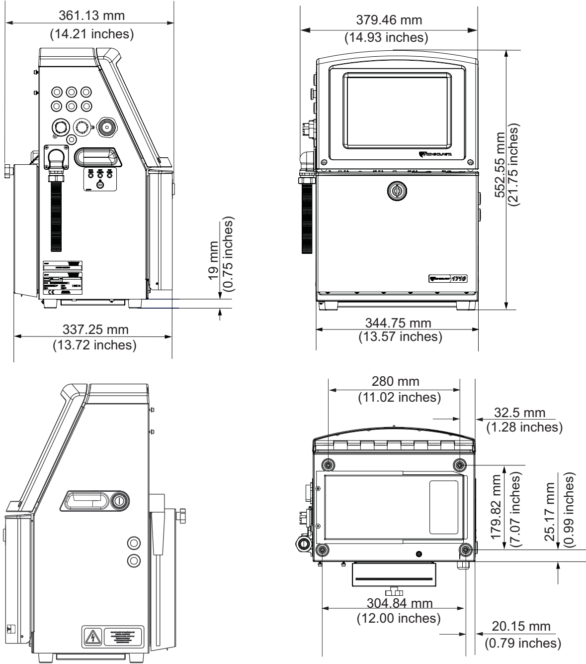
Şekil A-1: Yazıcı Ölçüleri
