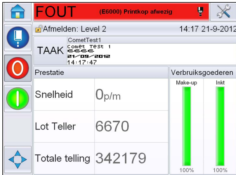
Afbeelding 7-5: Storingsweergave
