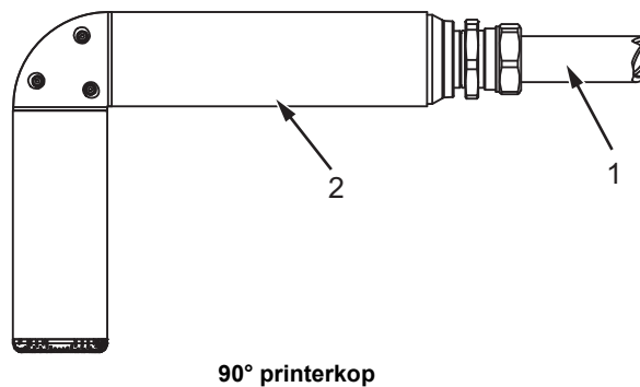
Afbeelding 3-7: Printkop en voedingsleiding
