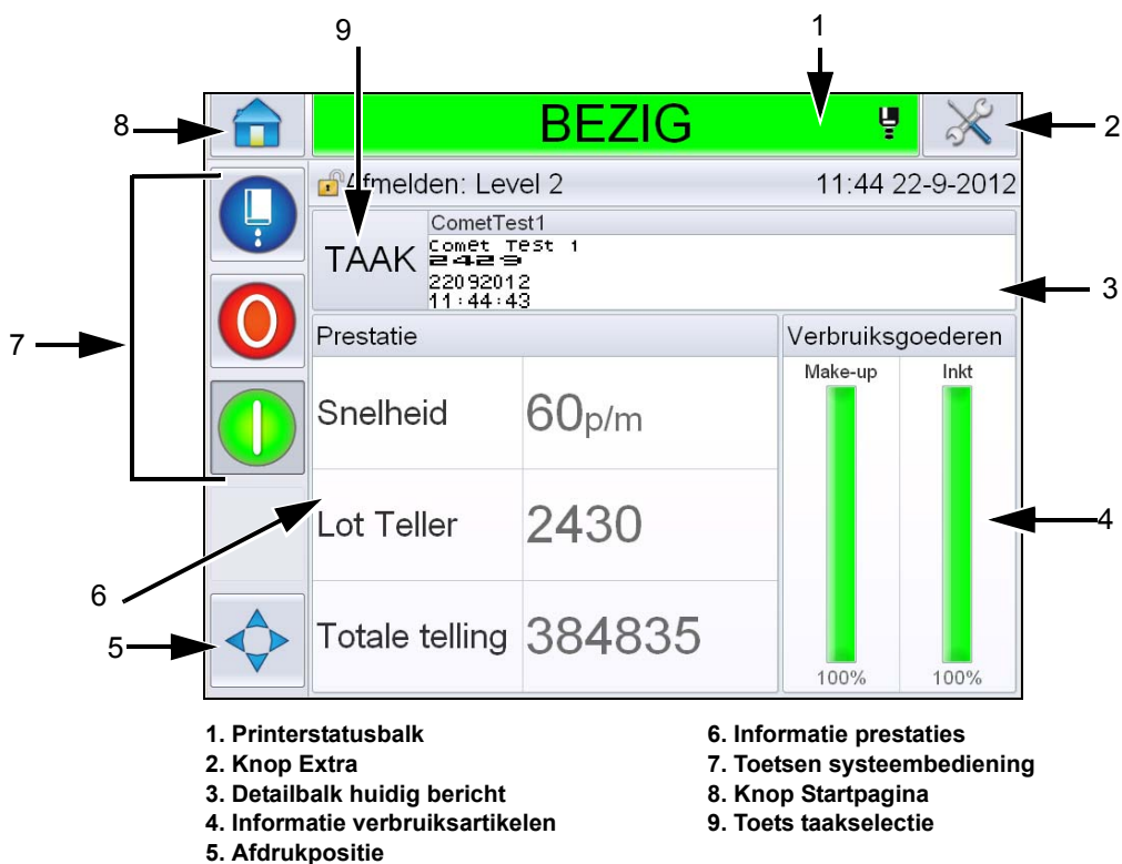
Afbeelding 5-1: Startpagina
