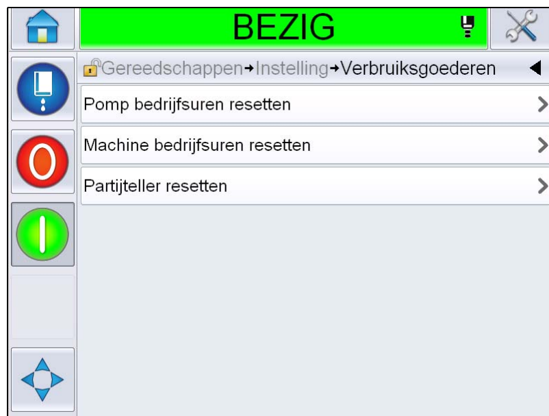
Afbeelding 4-8: Tellers terugzetten
