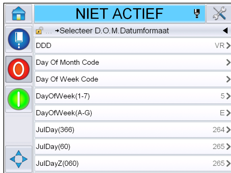
Afbeelding 5-27: Pagina datumformaat
