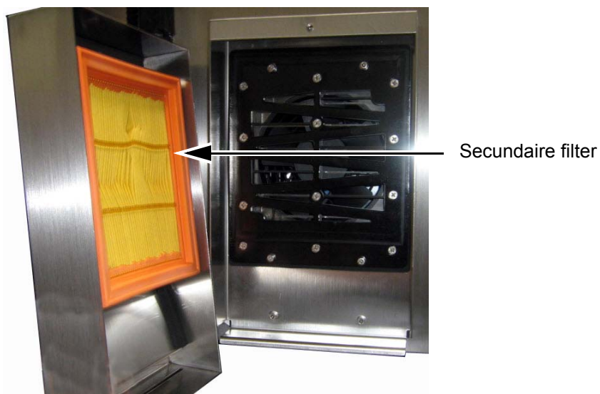
Afbeelding 3-11: Secundaire filter (IP65-versie)
