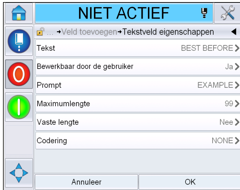
Afbeelding 5-58: Tekstveldeigenschappen
