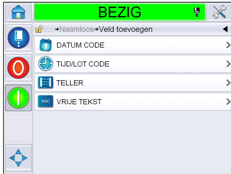
Afbeelding 5-24: Veld toevoegen
