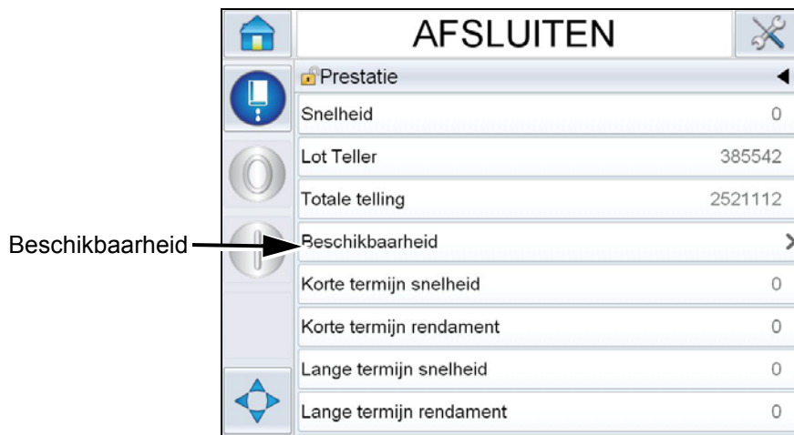
Afbeelding 5-66: Pagina prestaties
