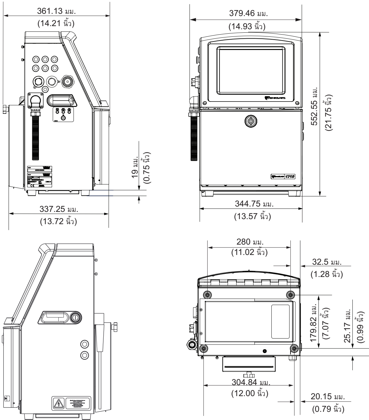
ภาพ A-1: ขนาดเครื่องพิมพ์
