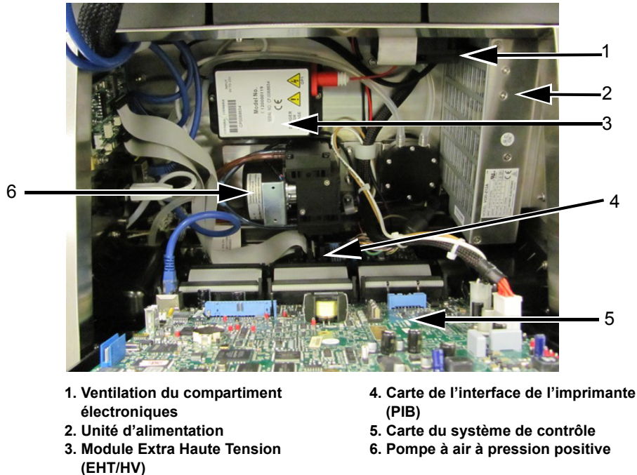
Figure 3-4 : Compartiment électronique
