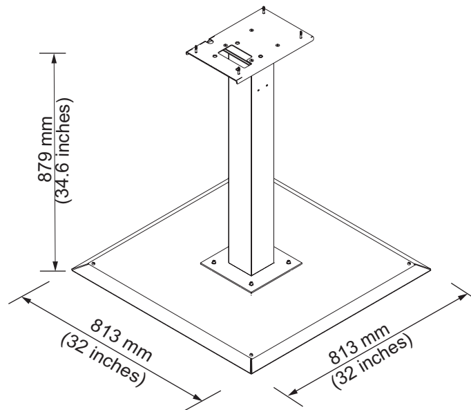
Figure A-3 : Support d'imprimante fixe
