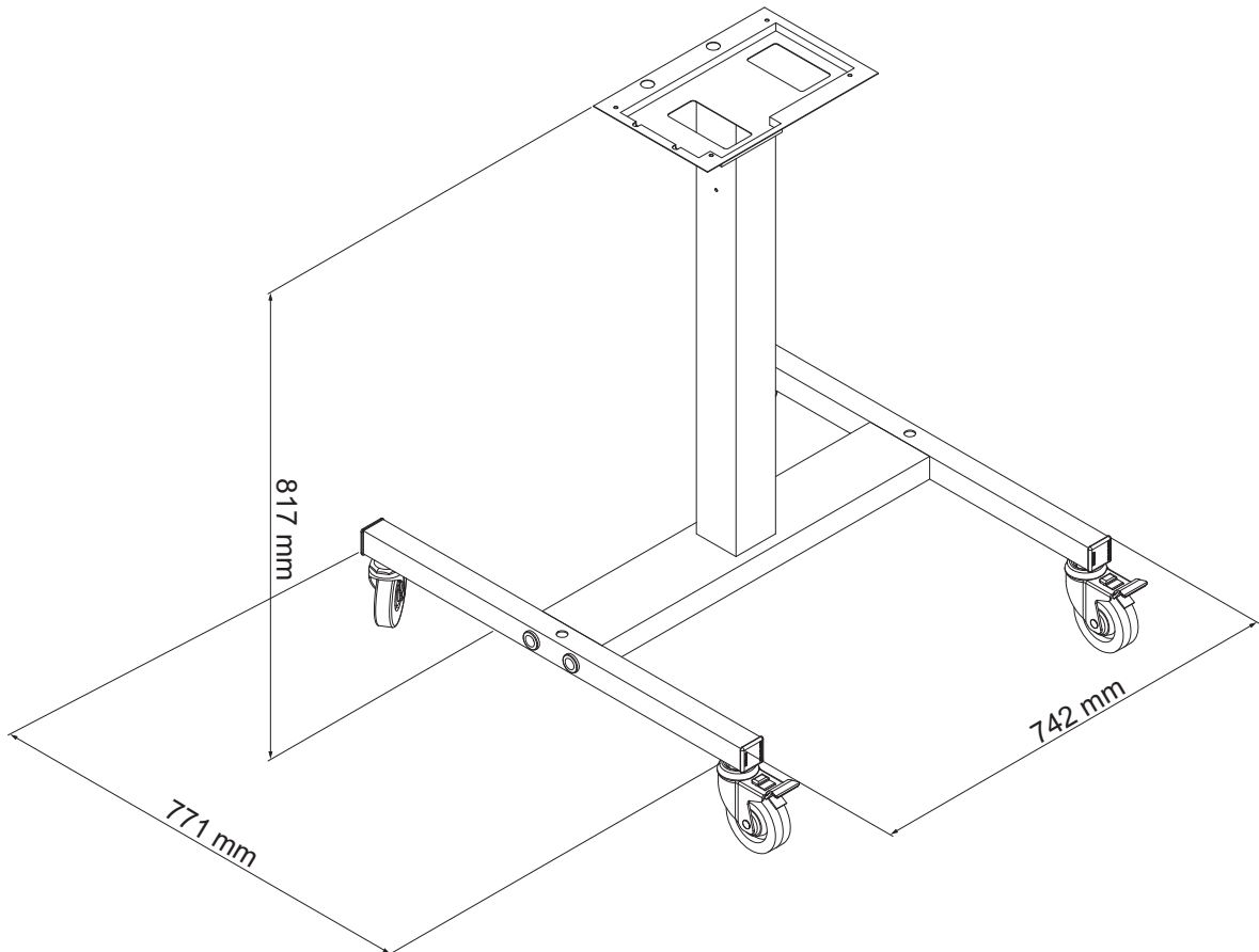
Figure A-3: Dimensões do suporte móvel da impressora
