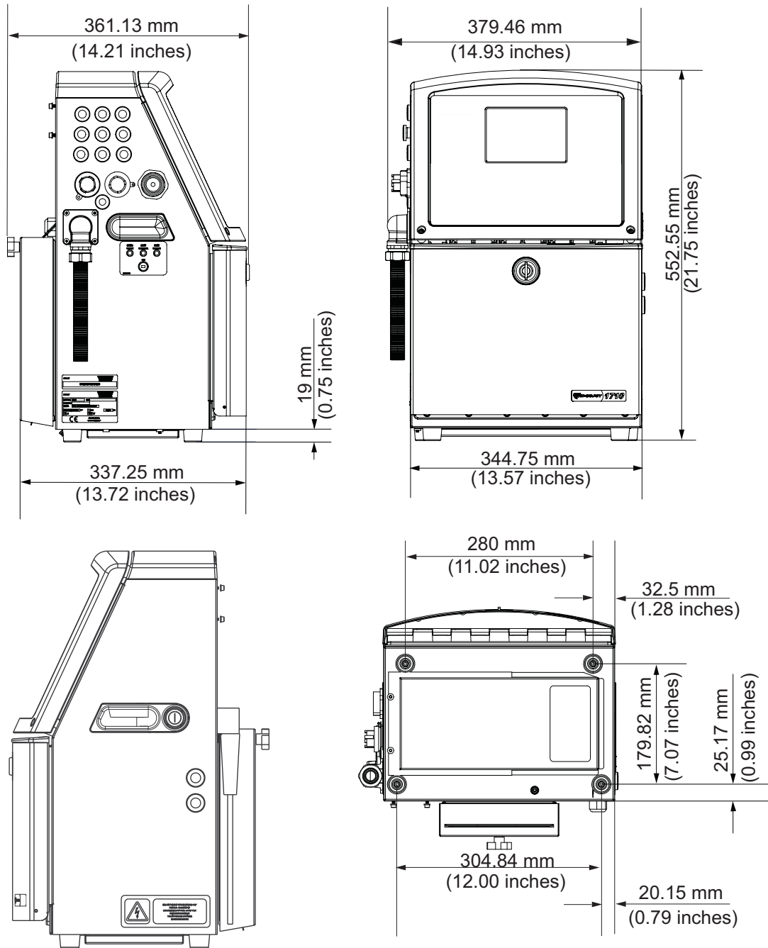
Figura A-1: Dimensões da impressora
