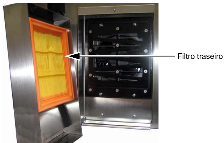
Figura 3-11: Filtro traseiro (versão IP65)
