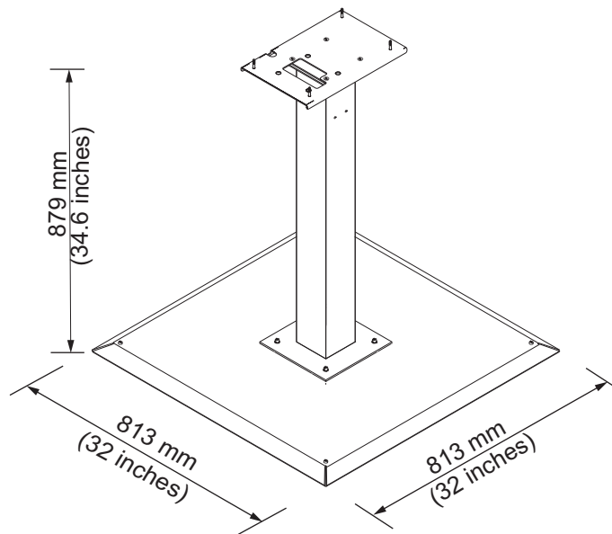
Figura A-4: Suporte Fixo da Impressora
