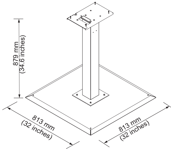
Afbeelding A-4: Statisch Printer Statief
