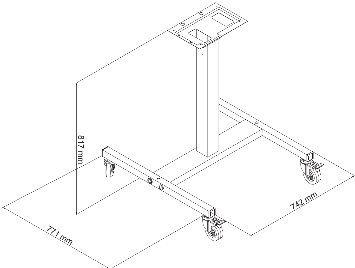
Figure A-3: Afmetingen mobiel printerstatief
