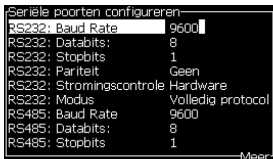
Afbeelding 4-21: Dialoogvenster Seriële poorten configureren
