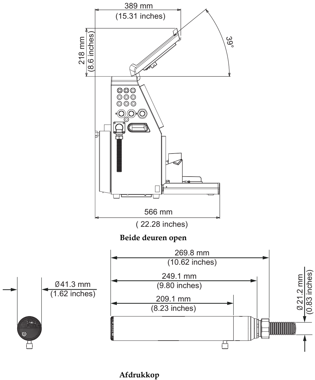
Afbeelding A-2: Printerafmetingen
