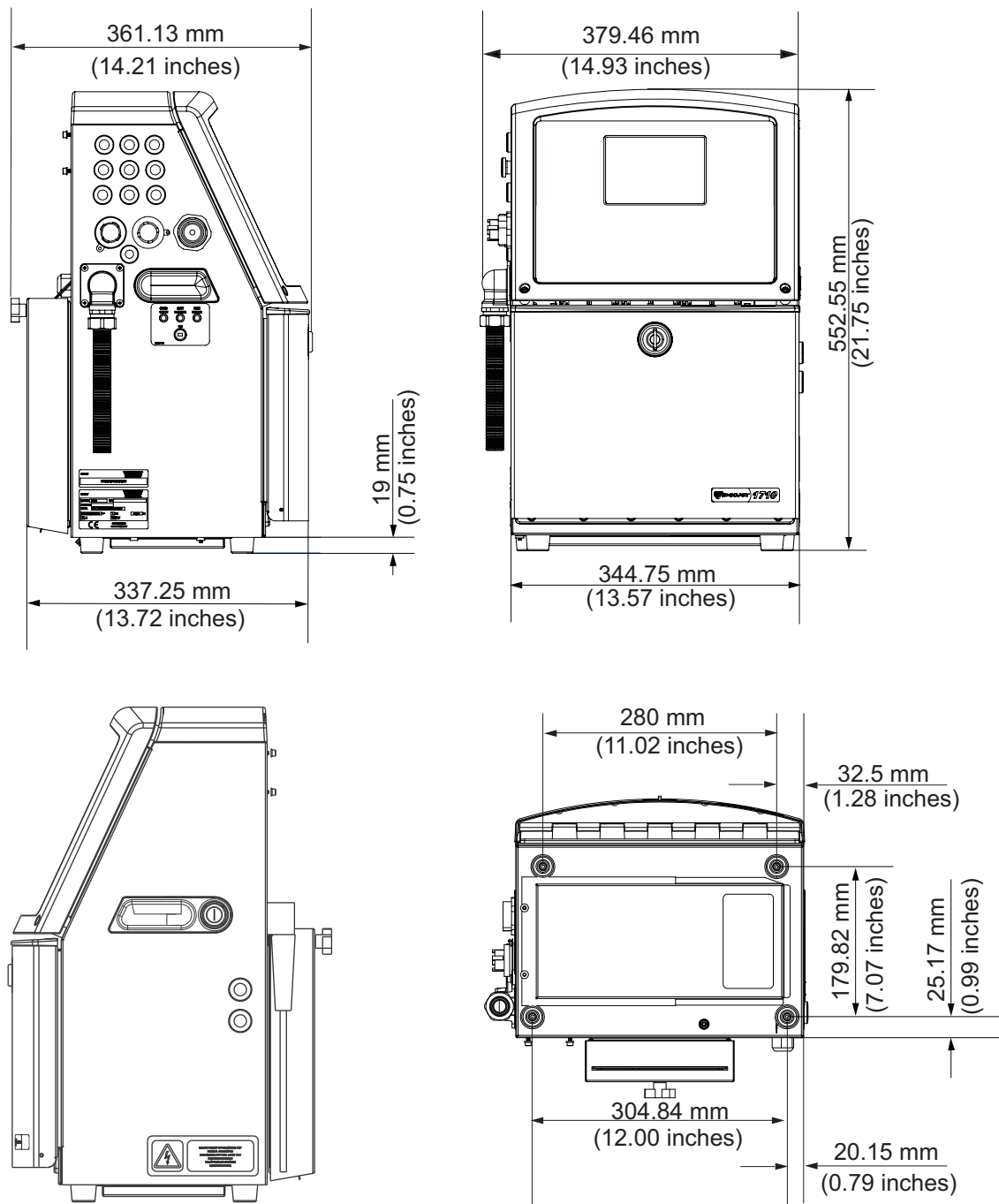
Afbeelding A-1: Printerafmetingen
