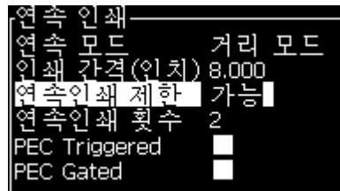
그림 4-28: 거리 모드
