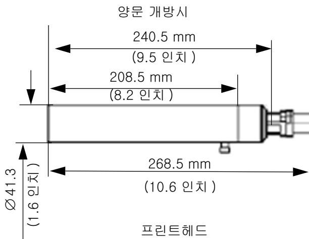
그림 A-3: 프린터 크기 Videojet 1220 ( 계속 )
