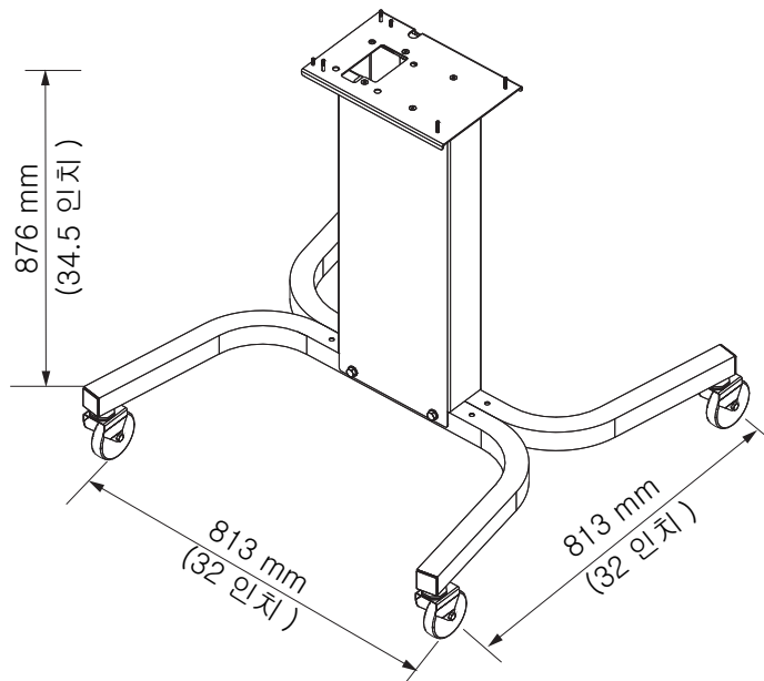
그림 A-5: 이동용 프린터 스탠드
