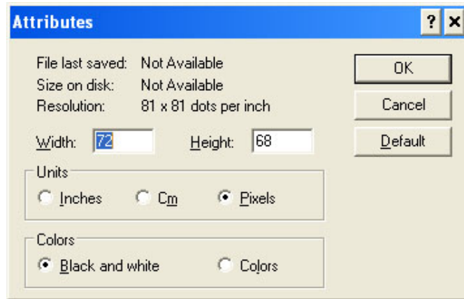
그림 5-44: 이미지 속성
