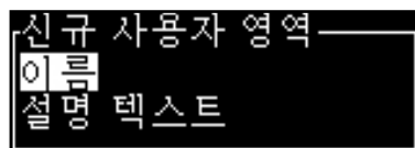
그림 5-23: 텍스트 속성
