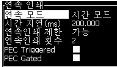
그림 4-27: 시간 모드
