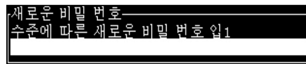
그림 4-5: 새 비밀번호
