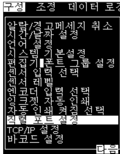
그림 4-19: 구성 메뉴
