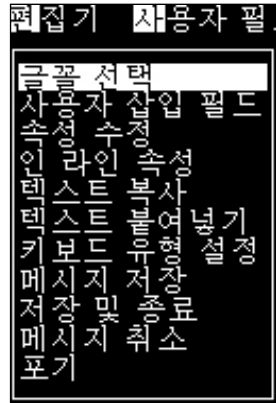
그림 5-33: 편집기 메뉴
