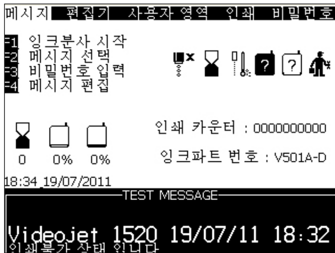
그림 1-1: 메뉴 화면
