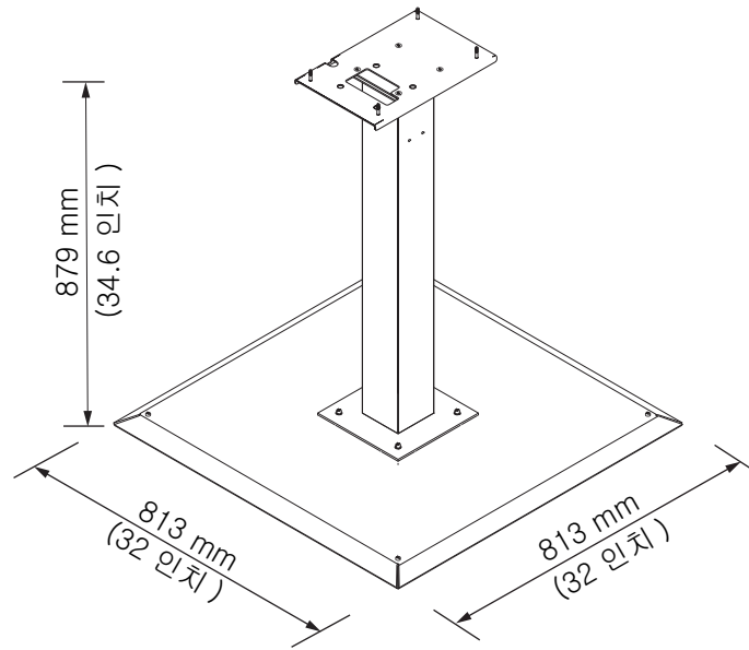
그림 A-6: 고정용 프린터 스탠드
