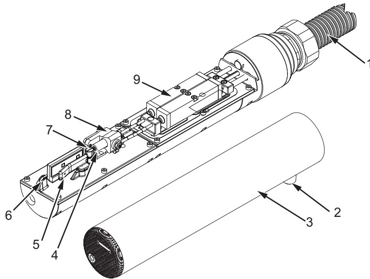
그림 6-4: 프린트헤드 (Videojet 1220)
