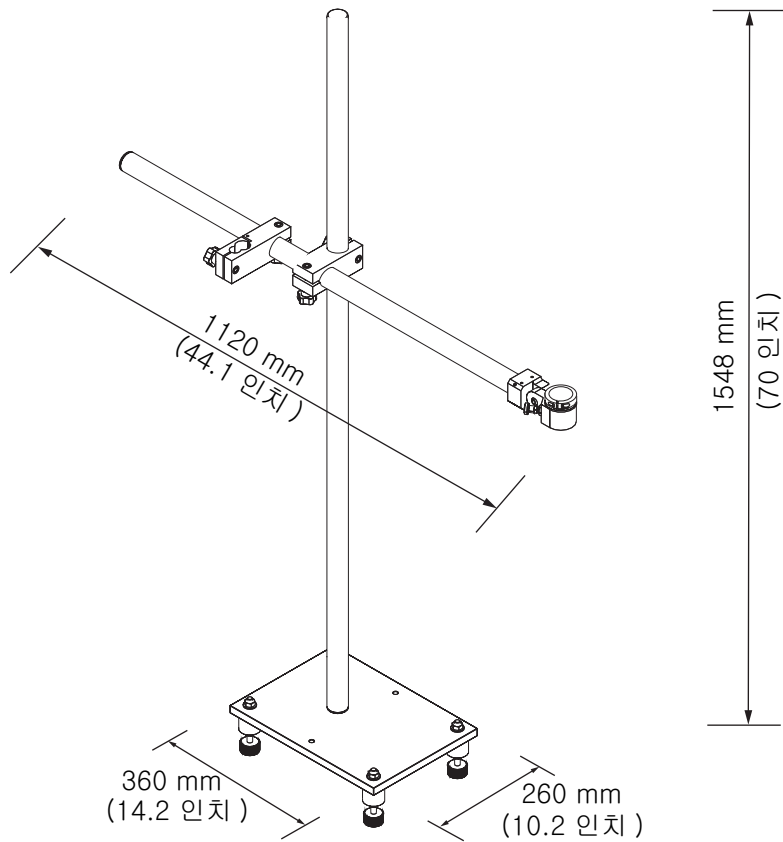
그림 A-7: 프린트헤드 스탠드
