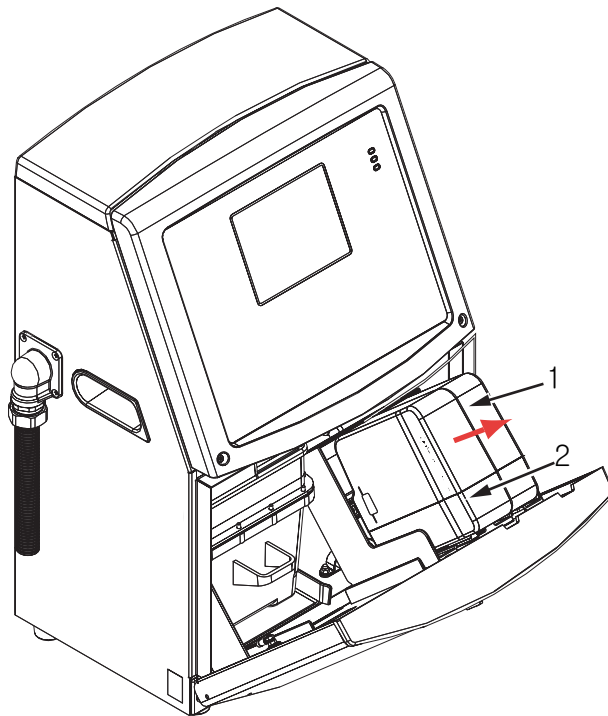
그림 6-2: 카트리지를 잡아 당기기
