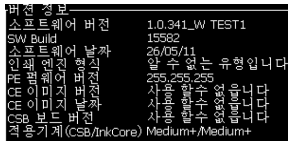
그림 4-15: 버전 정보
