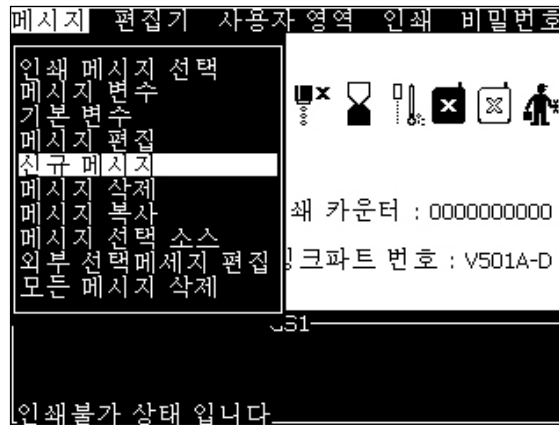
그림 5-3: 메시지 메뉴
