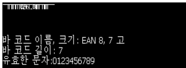
그림 5-41: 바 코드
