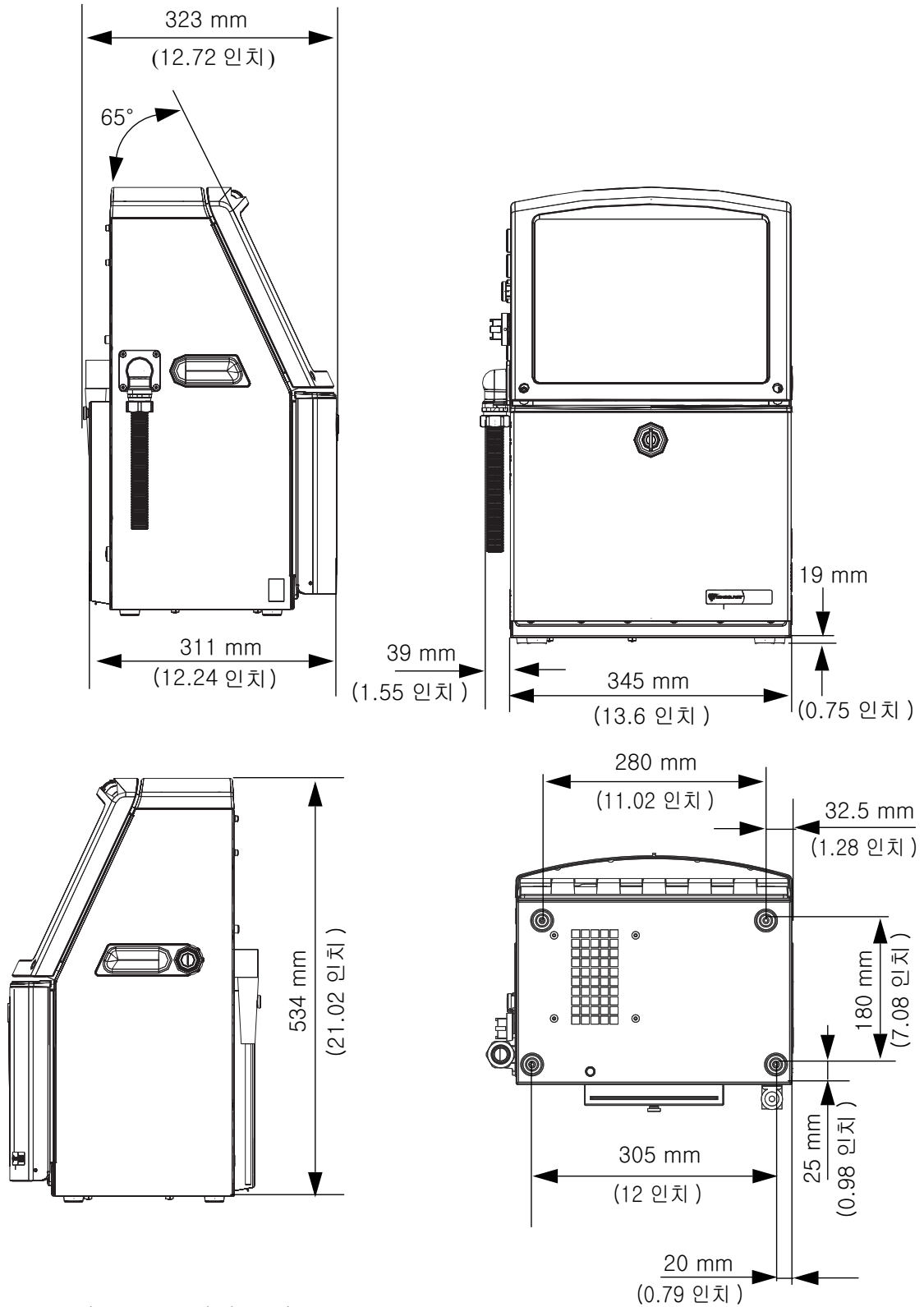
그림 A-1: 프린터 크기 Videojet 1220
