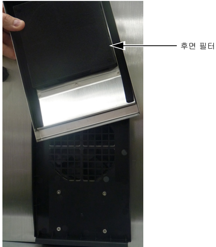
그림 3-14: 후면 필터 (IP55 버전 ) - Videojet 1220
